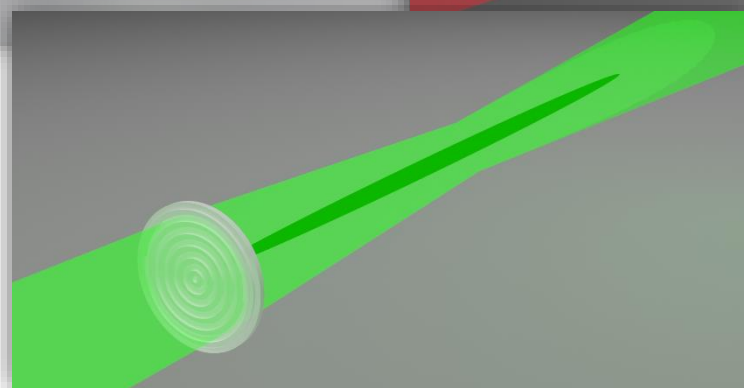
Bessel beam
